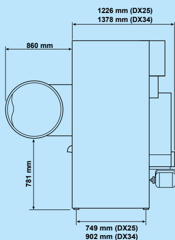
Parte lateral DX25 34
