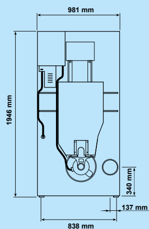
Parte trasera DX25 34 El.
