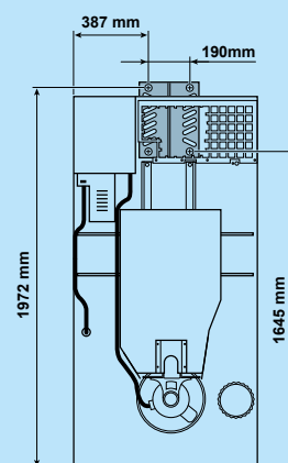
Parte trasera DX25 34 Vapor
